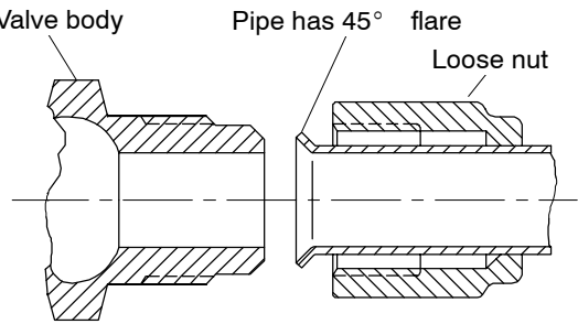
Fig. 15. 1/2" flare
